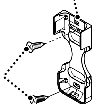
Skrutky na pripevnenie držiaka diaľkového ovládača
